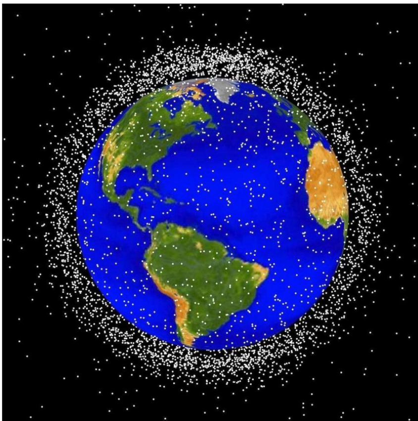
Rămășițe în spațiul cosmic Sursa: Internet
