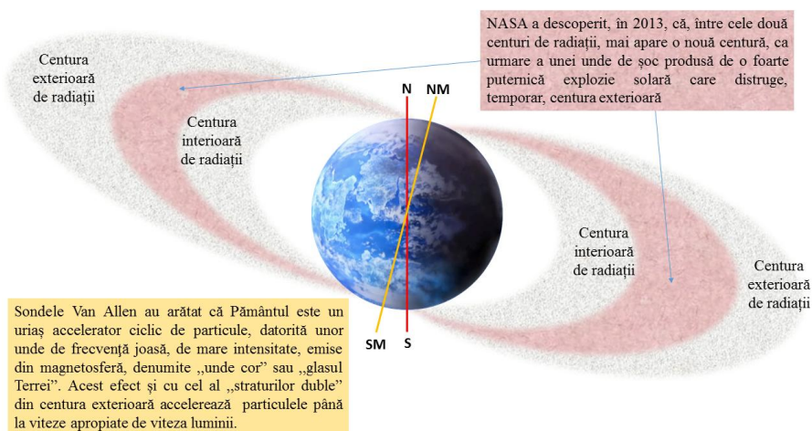
Figura nr. 1 Centurile de radiații Van Allen
